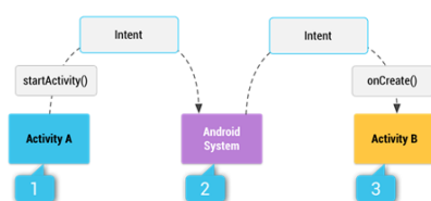
Figura 1: Ilustración de la forma en que se entrega una intent implícita mediante el sistema para iniciar otra actividad. [1] La actividad A crea una Intent con una descripción de acción y la pasa a startActivity() . [2] El sistema Android busca en todas las apps un filtro de intents que coincida con la intent. Cuando se encuentra una coincidencia, [3] el sistema inicia la actividad coincidente ( actividad B ) invocando su método onCreate() y pasándolo a la Intent . Fuente: Android Developer.
